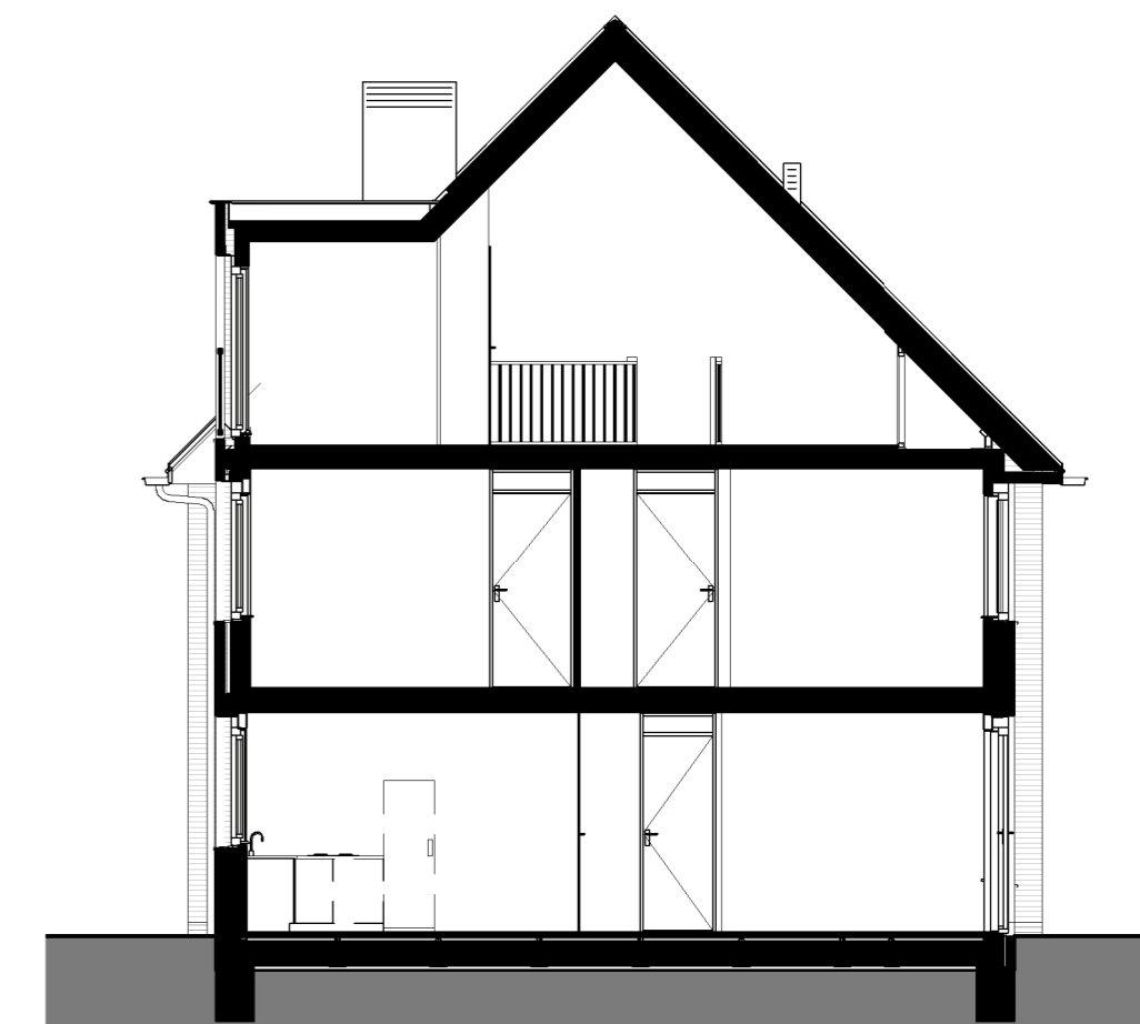
Dwarsdoorsnede A-A
