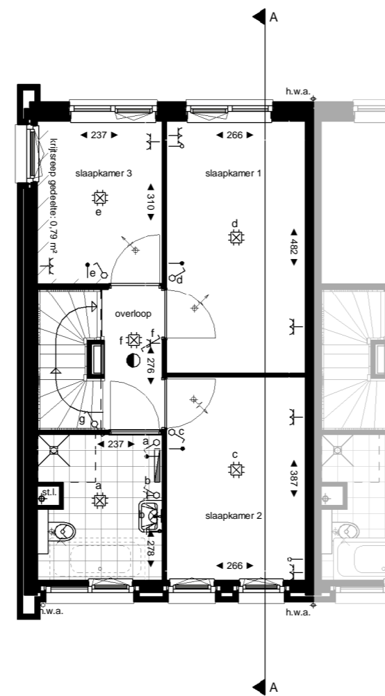
Eerste verdieping
