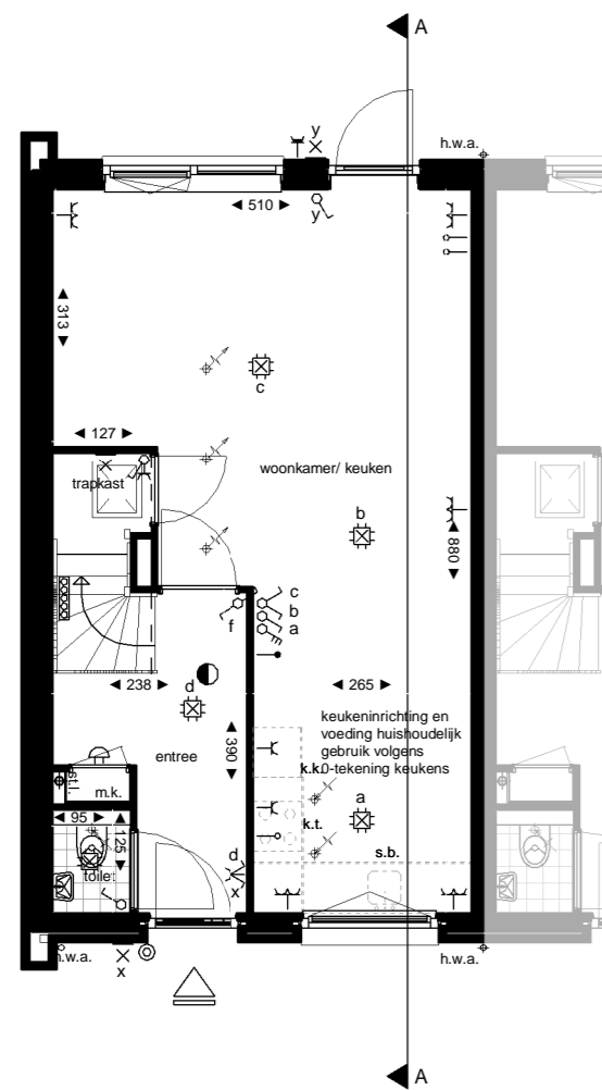
Begane grond
