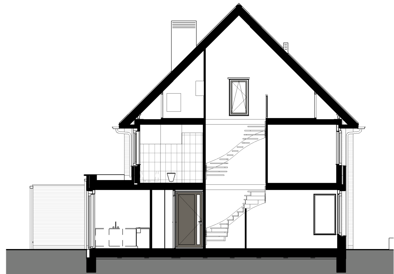
doorsnede A-A
