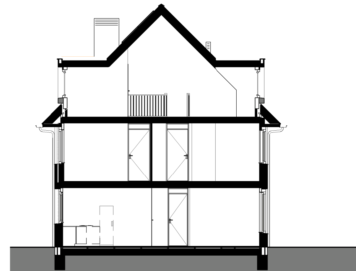
Dwarsdoorsnede A-A
