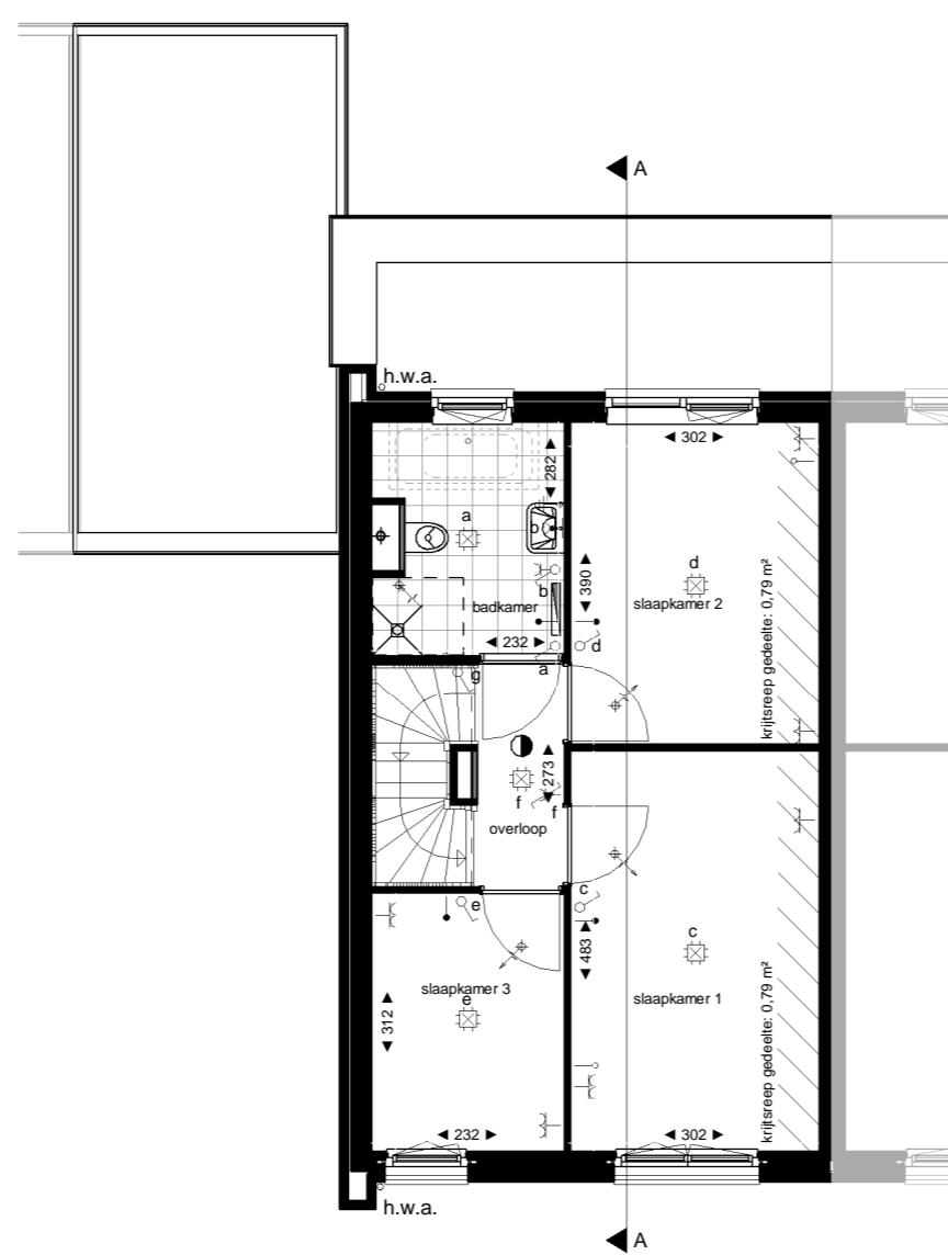
Eerste verdieping
