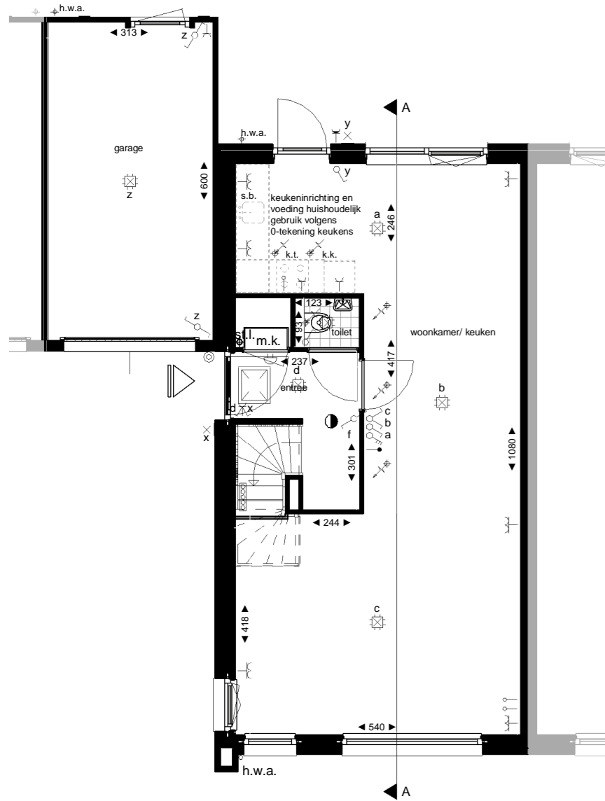
Begane grond
